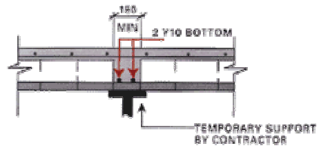
Stiffener Rib
